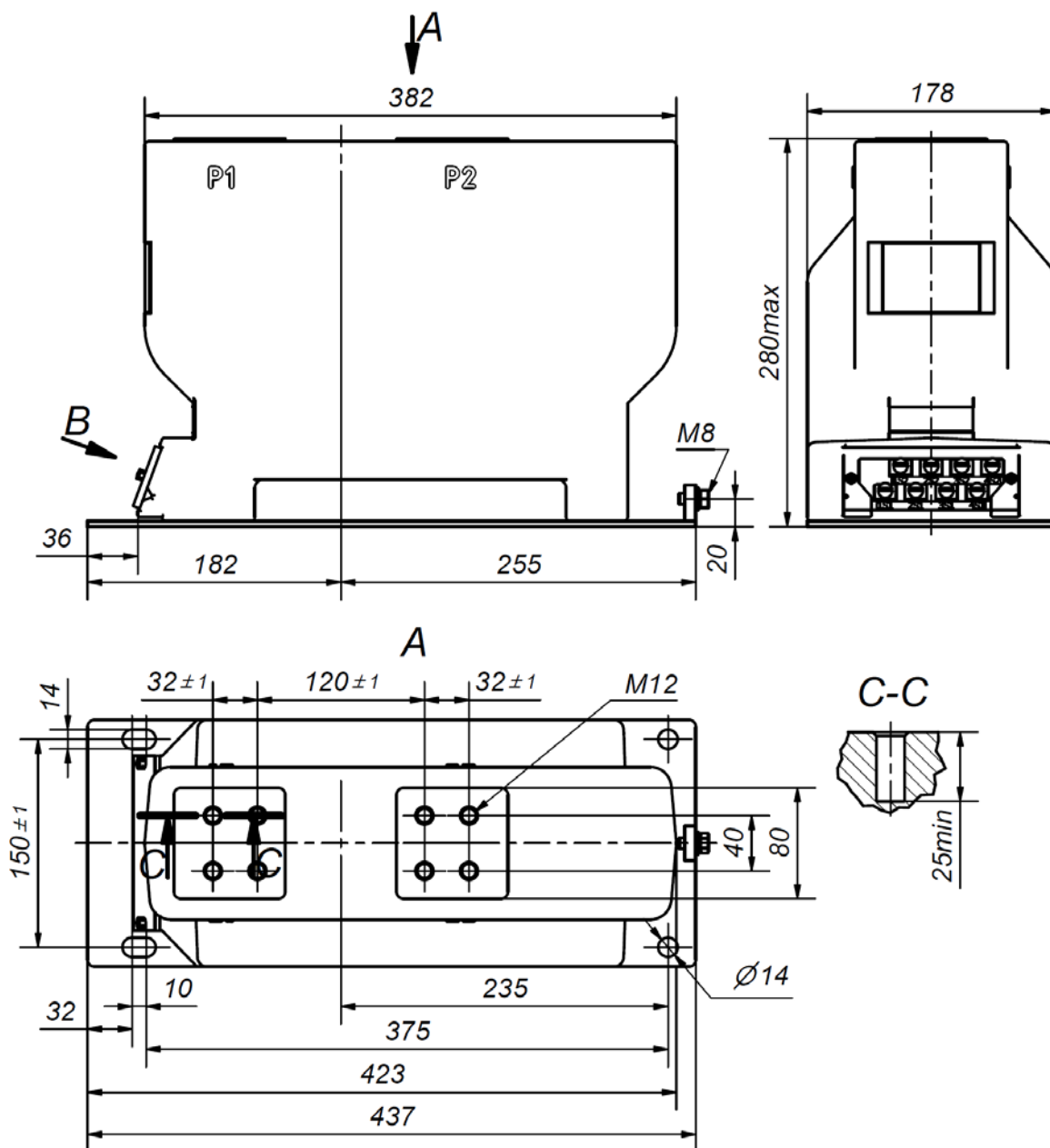
Рисунок А.3 Габаритне креслення трансформаторів TCS1-12-23.XX.2...
